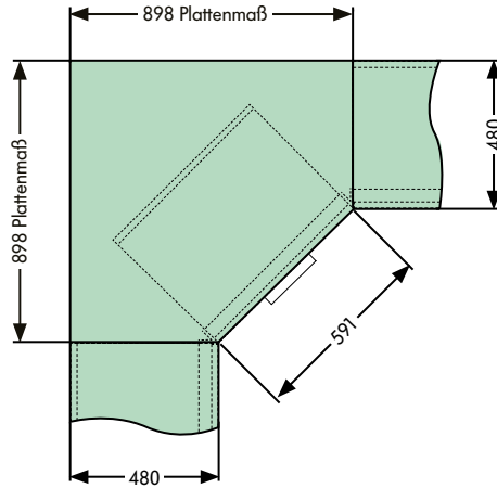
Ecklösung 135° mit Schrank 600 mm Breite und Blenden 400.0317.0 bzw. 400.0314.0 / 400.0315.0
