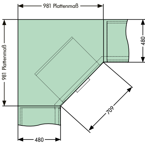
Ecklösung 135° mit Schrank 600 mm Breite und Blenden 400.0305.0
