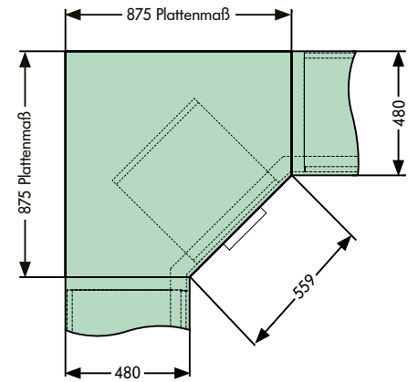
Ecklösung 135° mit Schrank 450 mm Breite und Blenden 400.0305.0
