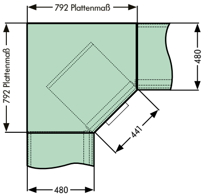
Ecklösung 135° mit Schrank 450 mm Breite und Blenden 400.0317.0 bzw. 400.0314.0 / 400.0315.0
