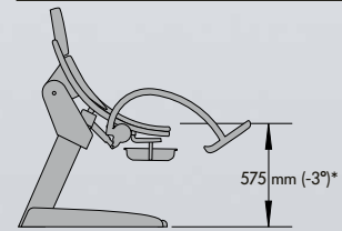
Gerade geformtes Sitzprofil für eine entspannte und fachgerechte Untersuchungsposition.
